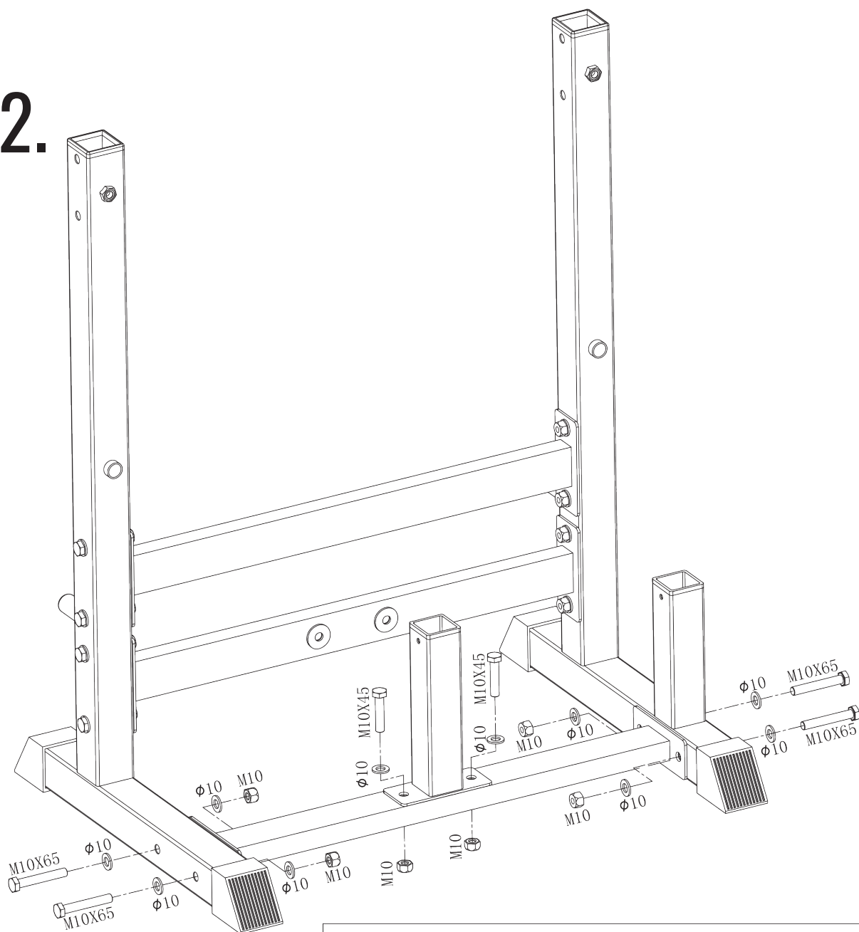
VIJAK (M10*65) X 4
