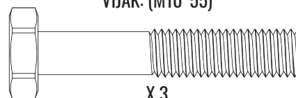
VIJAK: (M10*55)
