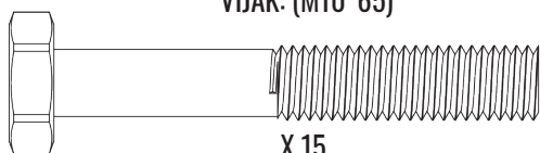
VIJAK: (M10*65)
